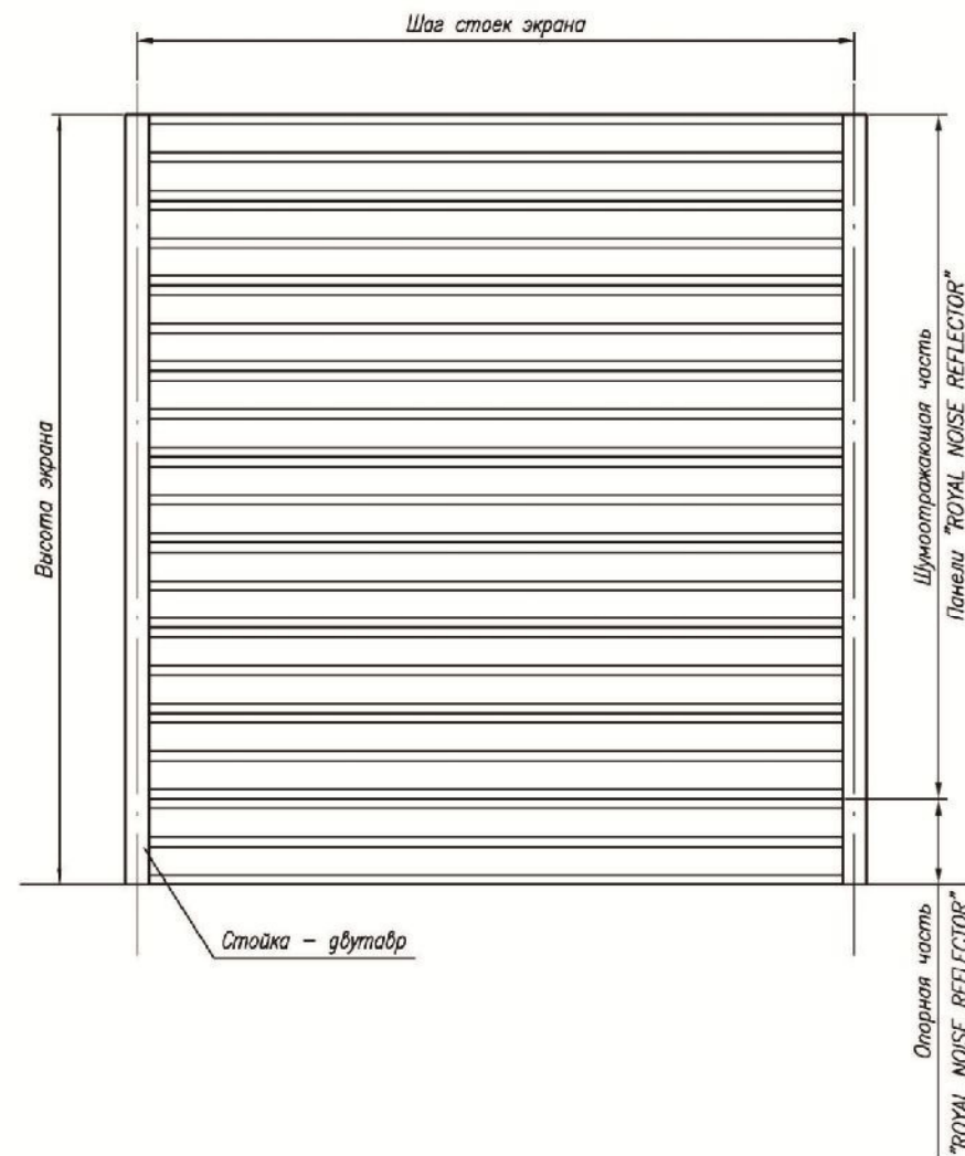
Экран шумоотражающий прямой непрозрачный
