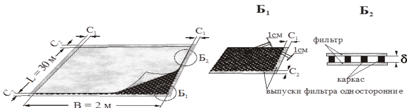
Рисунок А1 – Общая структура геодрены
