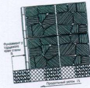
Рисунок 30 - Удлинение фундамента у края стены
