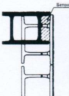
Рисунок 23 - Вариант заделки торца
