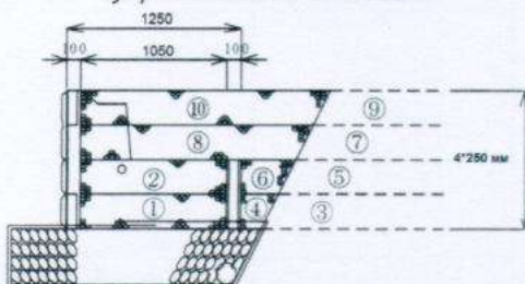
Рисунок 19 - Порядок уплотнения щебня для внутренней засыпки в короба и позади них у подпорной стены для насыпи, а также уплотнения самой
