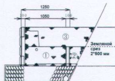
Рисунок 20 - Порядок уплотнения щебня для внутренней засыпки в короба и позади них у подпорной стены для земляного среза.
