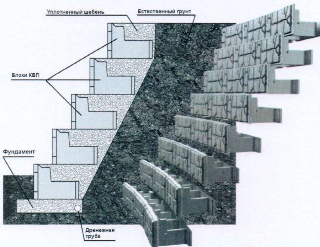
Рисунок 1 - Общий вид устройства подпорных стен
