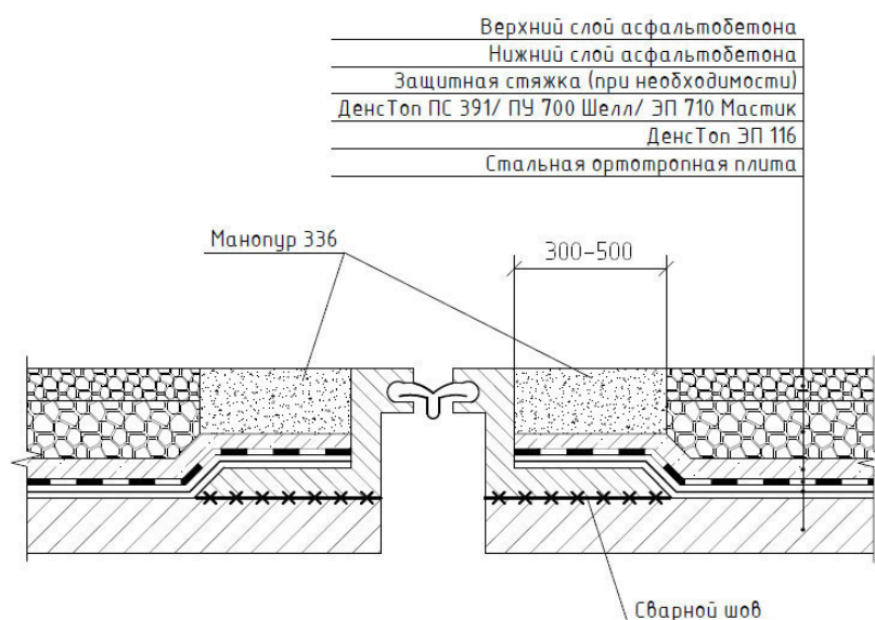
Рисунок 6.11 – Примыкание гидроизоляции к окаймлению конструкции деформационного шва с резиновыми компенсаторами (ортотропная плита)
