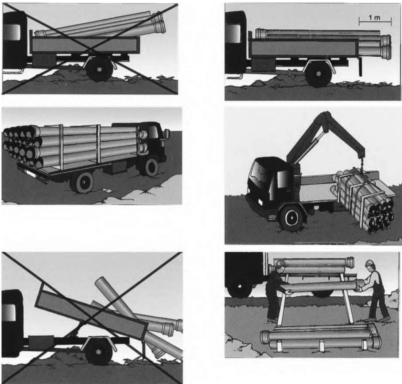
Рисунок 15 – Указание по транспортированию и перемещению труб
