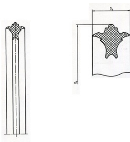
Рисунок 4 – Профиль резинового кольца
