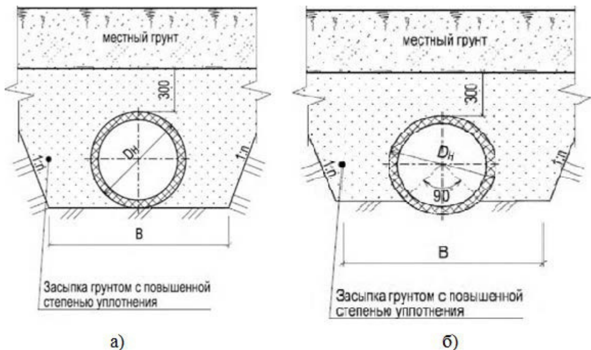
Рисунок 8 – Схема укладки труб, грунт основания: пески (кроме гравелистого)
