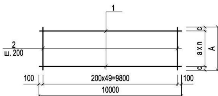
Рисунок Д. 1 – Конструкция арматурной сетки C1
