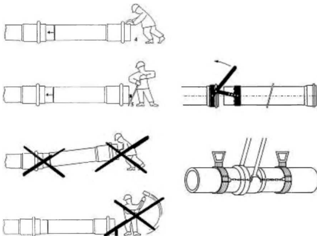
Рисунок 12 – Сборка раструбных соединений с уплотнительным кольцом
