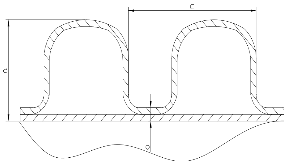
Рисунок 1 – Геометрические размеры гофрированной наружной поверхности
