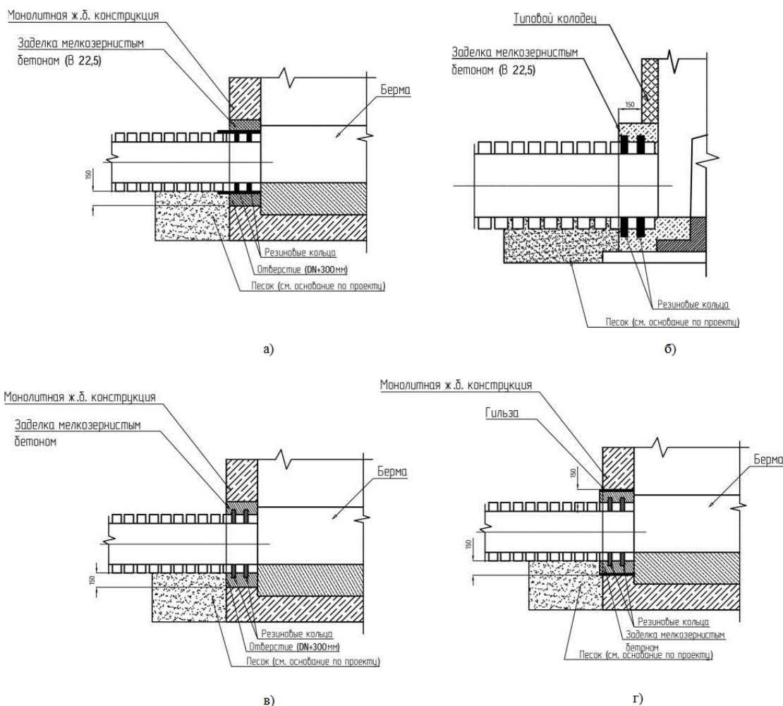
Рисунок 14 – Проход трубопровода через колодцы из железобетона: а), б), в) проход через колодец из монолитного железобетона, г) проход через типовой сборный бетонный колодец
