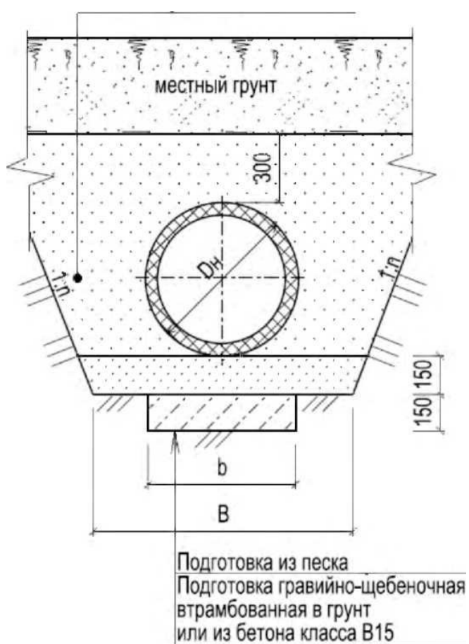
Рисунок 10 – Схема укладки труб, грунт основания: водонасыщенные грунты со слабой водоотдачей
