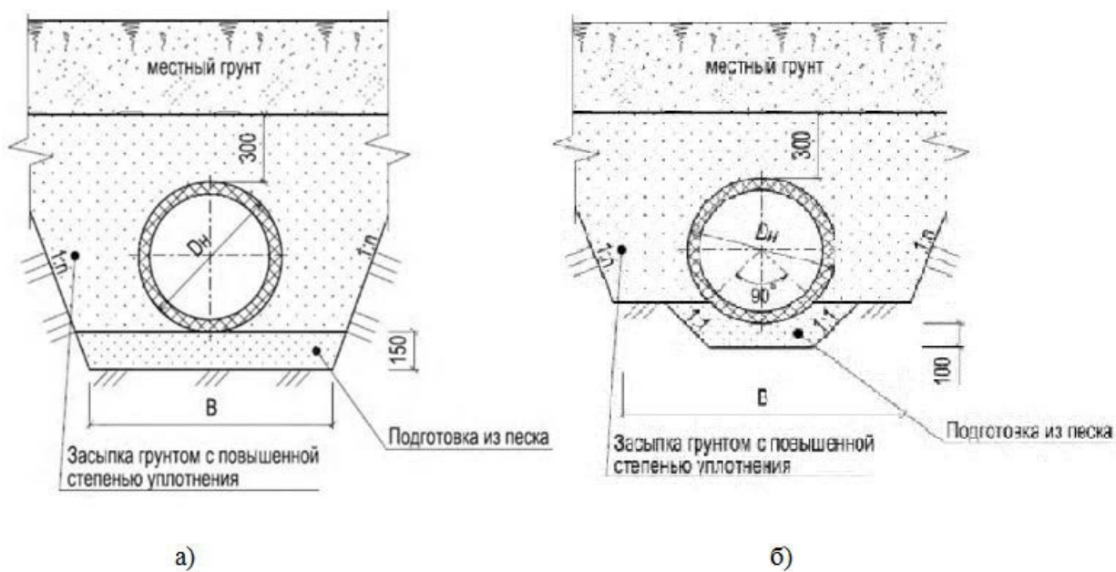
Рисунок 9 – Схема укладки труб, грунт основания: глинистые, гравелистые грунты, крупнообломочные скальные породы
