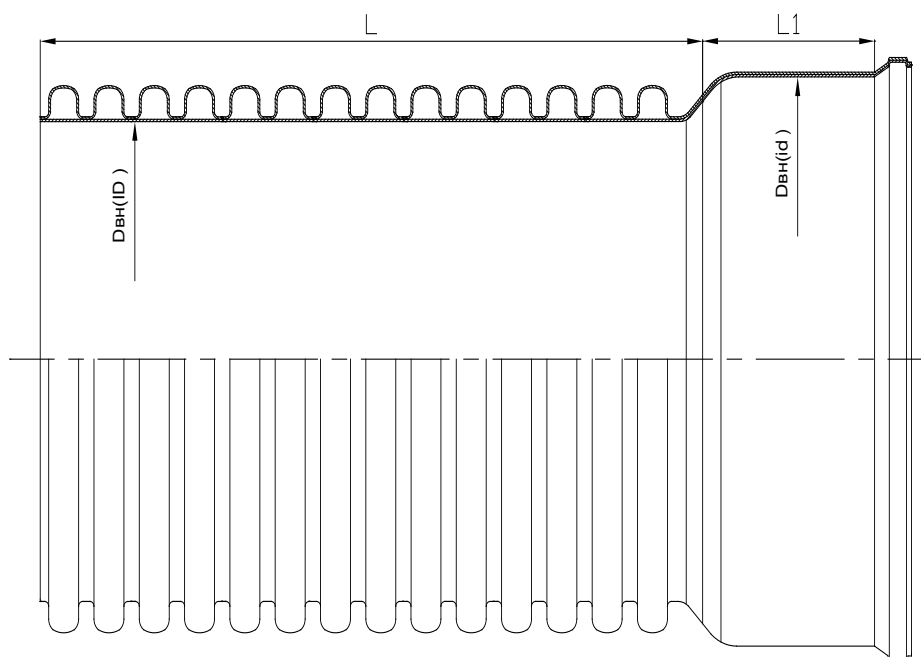
Рисунок 2 – Длина раструба
