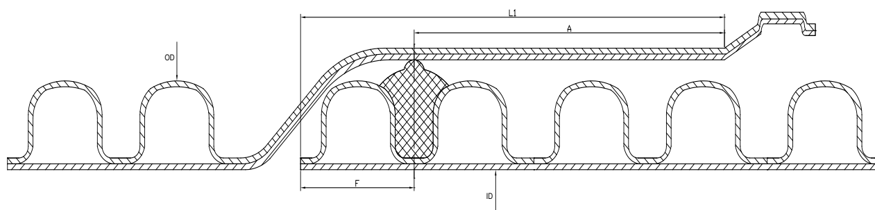
Рисунок 3 – Формирование раструба в процессе экструзии
