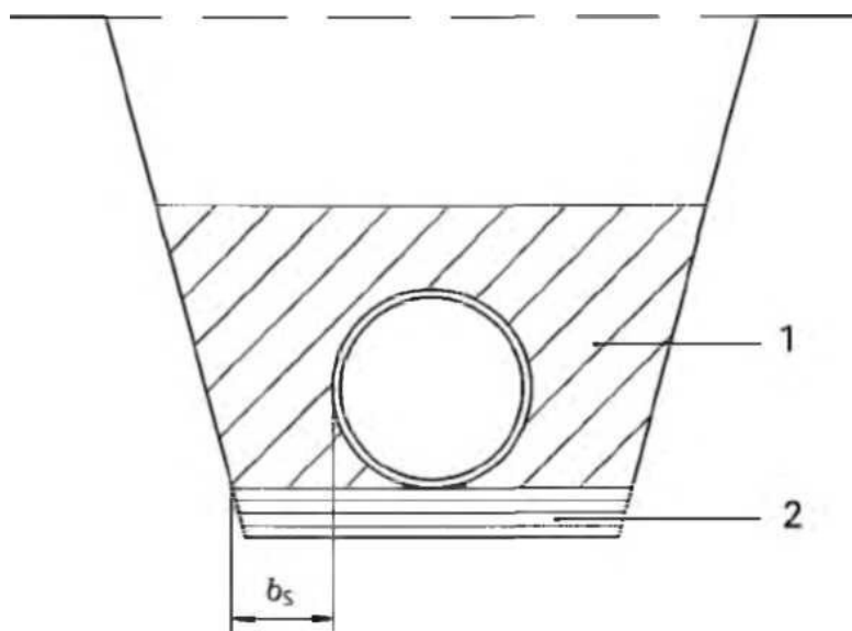
Рисунок 7 – Расстояния от трубы до стенки траншеи: 1 - засыпка в зоне трубы, 2 – основание
