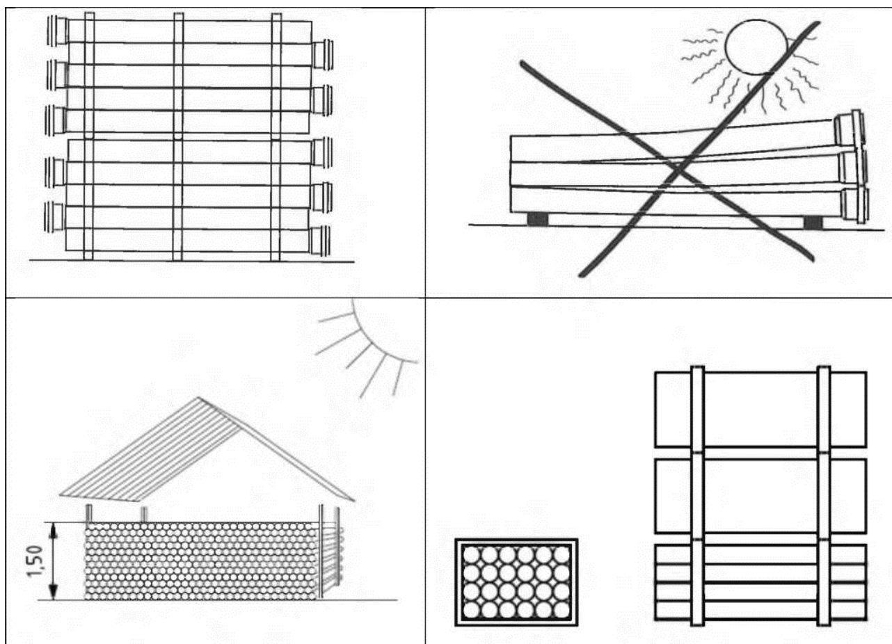
Рисунок 16 – Указания по хранению труб
