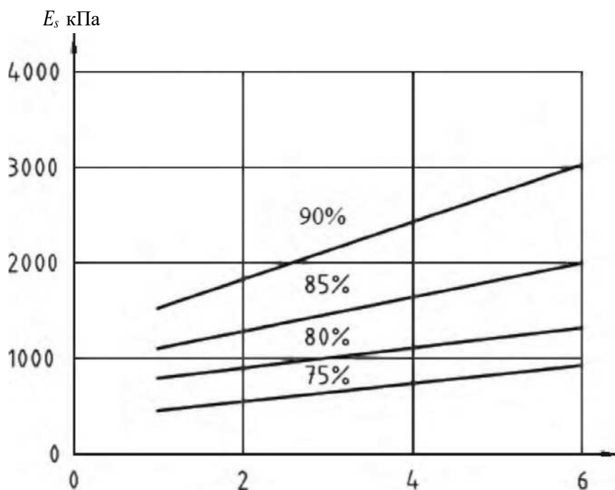
Рисунок 6 – Минимальные значения секущего модуля для несвязных грунтов
