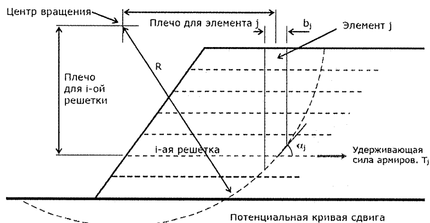
Рисунок А.7 - Цилиндрическая поверхность обрушения
