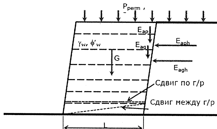
Рисунок А.5 - Расчетная схема для проверки на внутренний сдвиг
