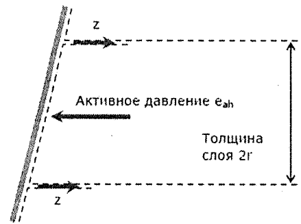
Рисунок А.6 - Проверка прочности облицовки
