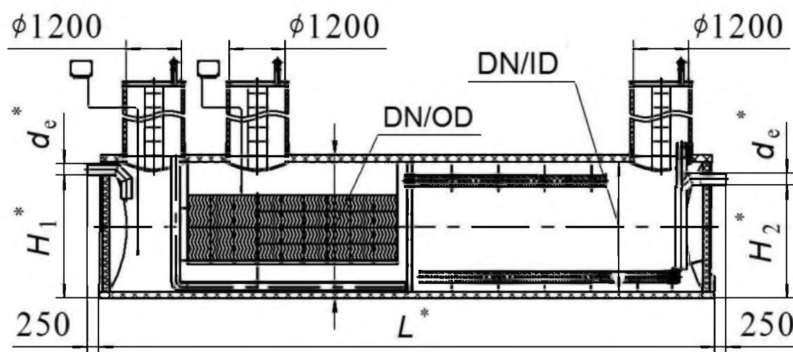
Рисунок 8 – Модифицированное очистное сооружение поверхностного стока (ПЕО-М/МБО/СОФ)
