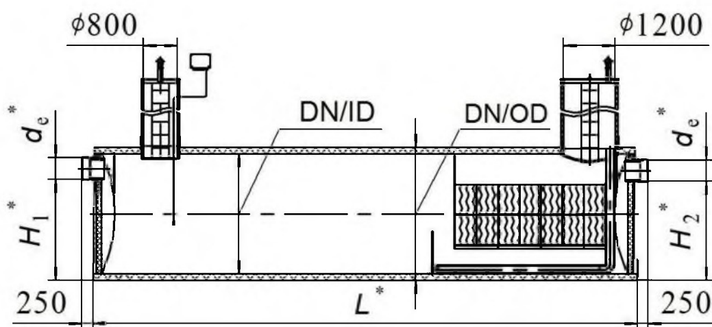
Рисунок 10 – Модифицированный пескоотделитель (ПЕО-М)
