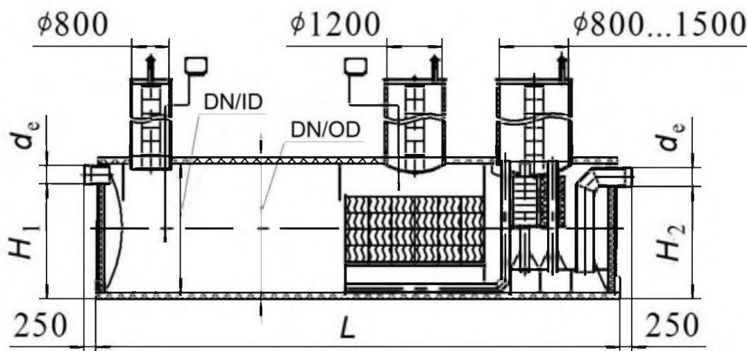
Рисунок 6 – Модифицированный пескомаслобензоотделитель (ПЕО/МБО-М)
