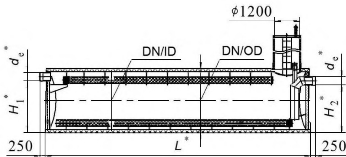
Рисунок 12 – Сорбционный фильтр (СОФ)
