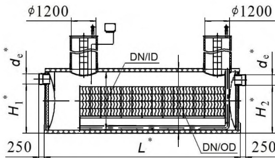
Рисунок 11 – Маслобензоотделитель (МБО)
