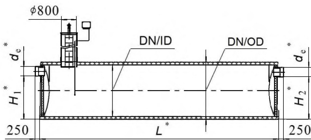
Рисунок 9 – Пескоотделитель (ПЕО)
