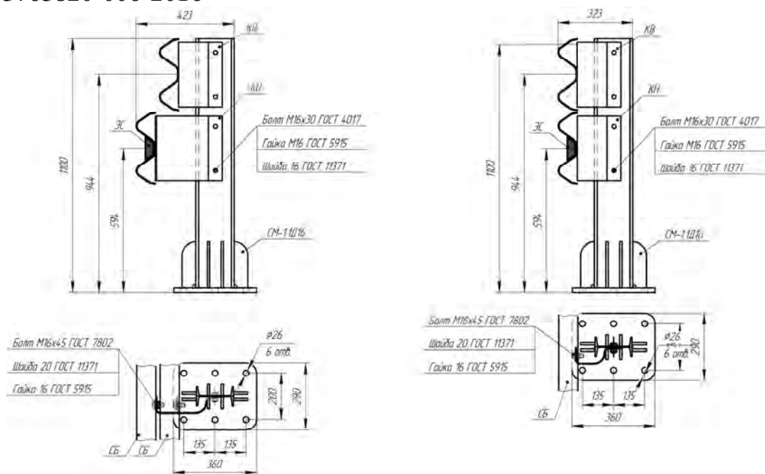
Рисунок В.69 - Мостовое ограждение 21МО/500÷600-1,1хS(Д16); 21МО/500÷600-1,1хS(Д16) без КН
