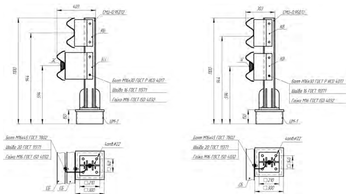
Рисунок В.35 - Ограждение мостовое 21МО/300÷450(Д12)Ц; 21МО/300-450(Д12)Ц без КН
