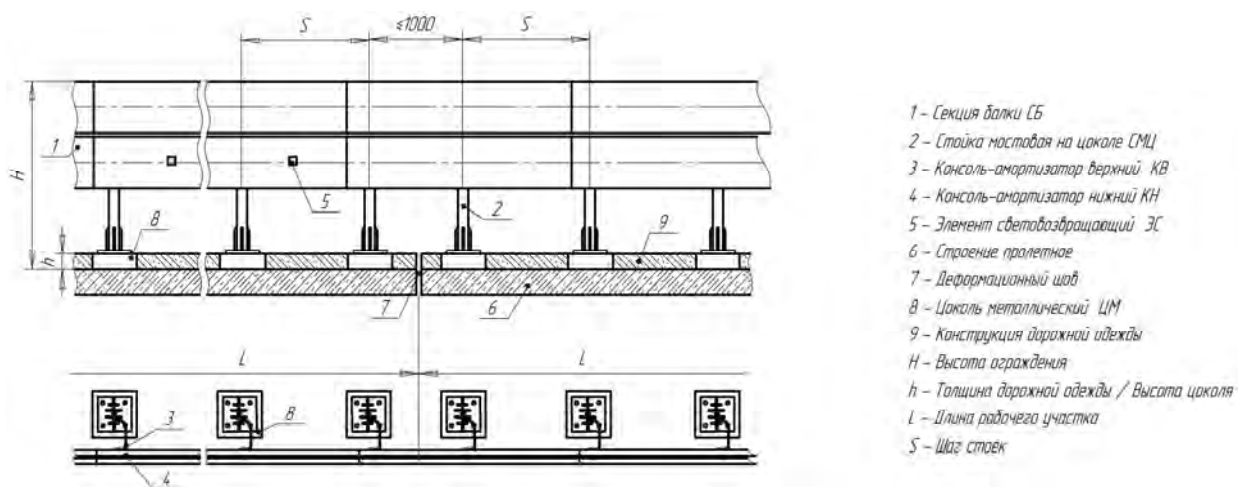
Рисунок В.9 - Ограждение группы 21МО/300-600(Ц)
