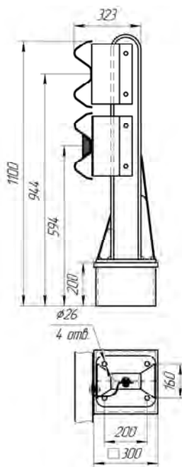
Рисунок 4.63 (СМЦ(1)-0,95Д16) без КН ЦМ-13
