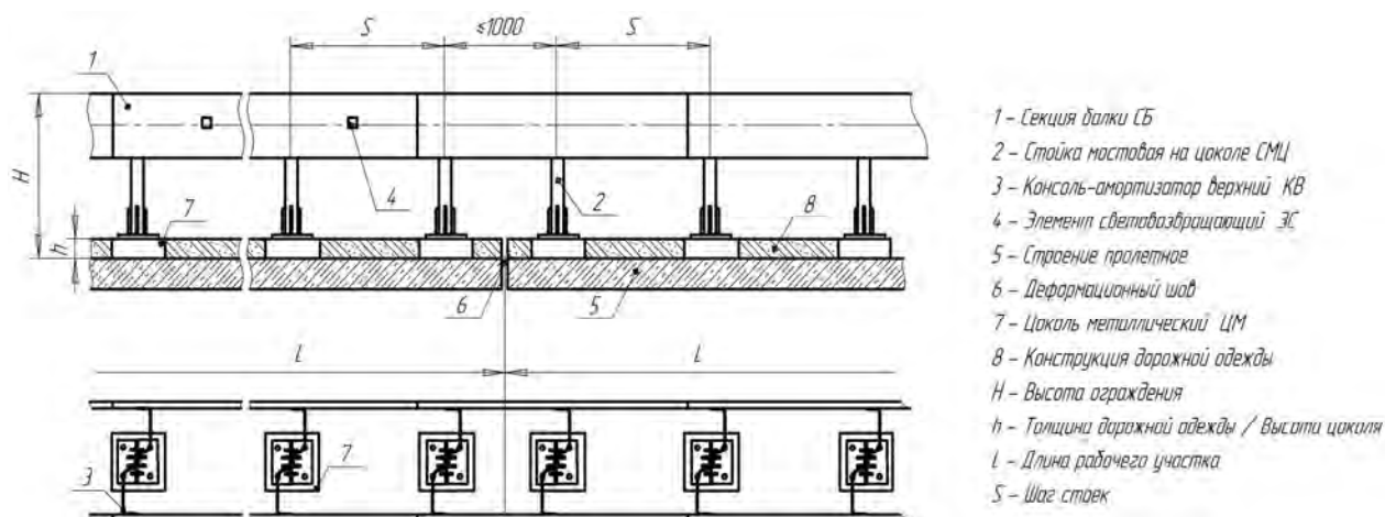
Рисунок В.8 - Ограждение группы 21МД/130-300(Ц)
