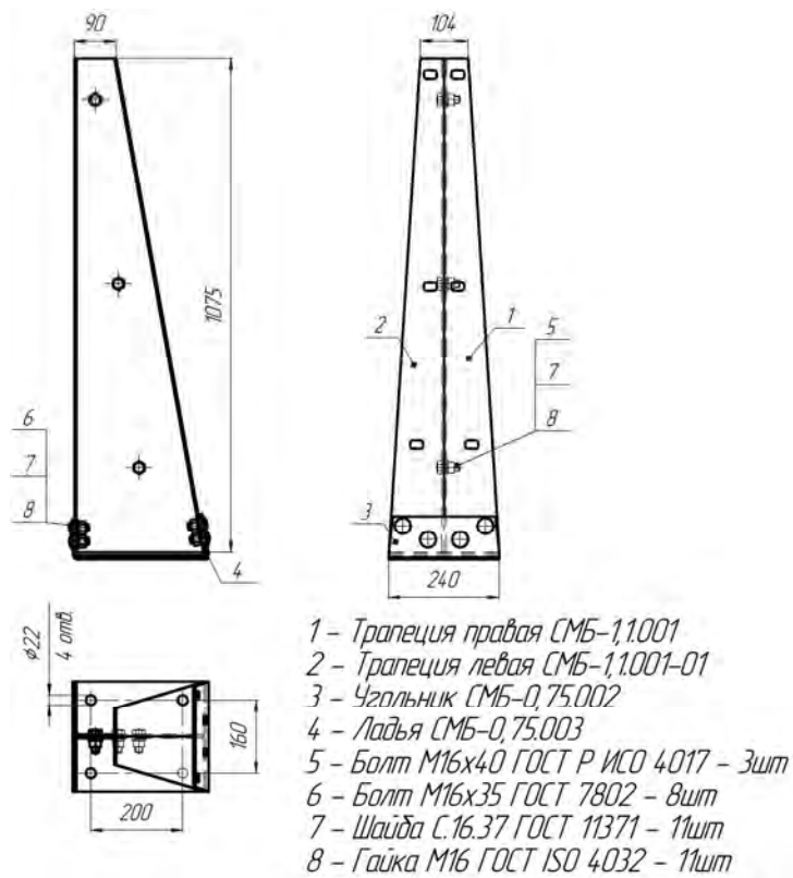
Рисунок В.29 - Стойка мостовая сборная СМБ-1,1
