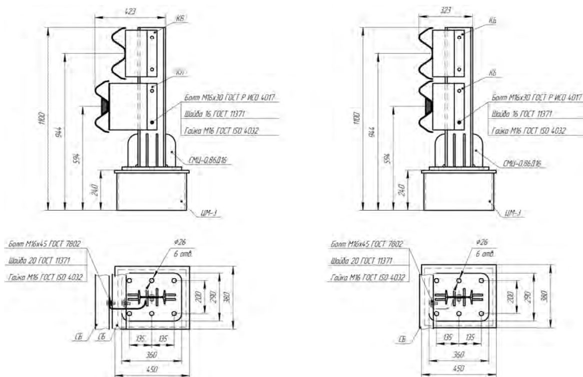
Рисунок В.70 - Мостовое ограждение 21МО/500÷600-1,1(Ц)хS(Д16); 21МО/500÷600-1,1(Ц)хS(Д16) без КН
