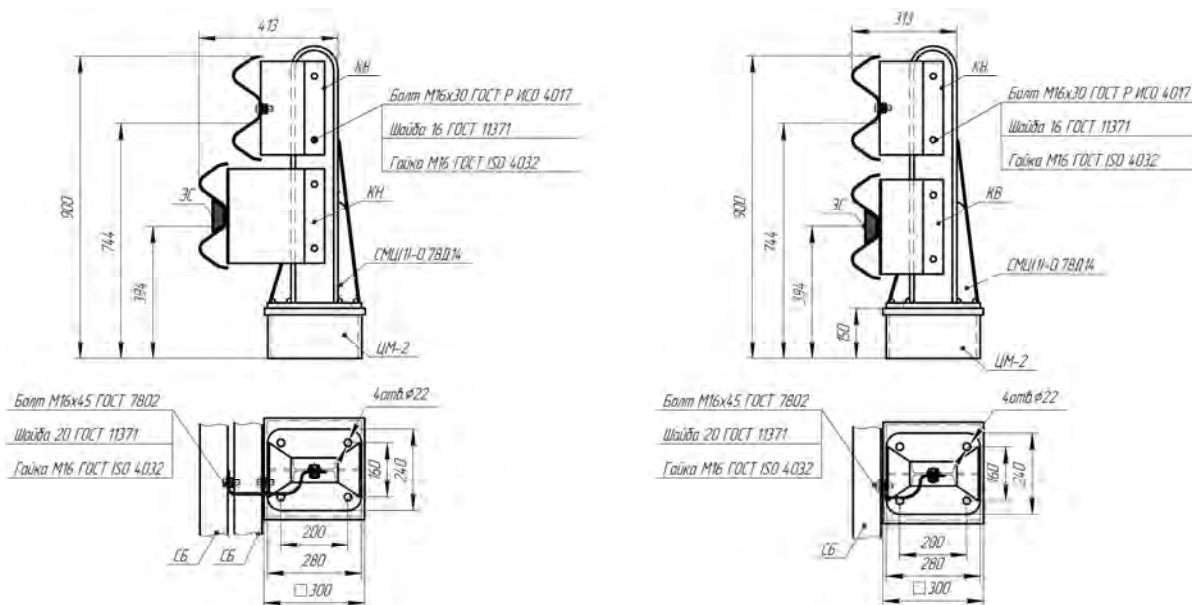
Рисунок В.51 – Мостовое ограждение 21МО/300÷450-0,9(Ц)хS(Д14); 21МО/300÷450-0,9(Ц)хS(Д14) без КН
