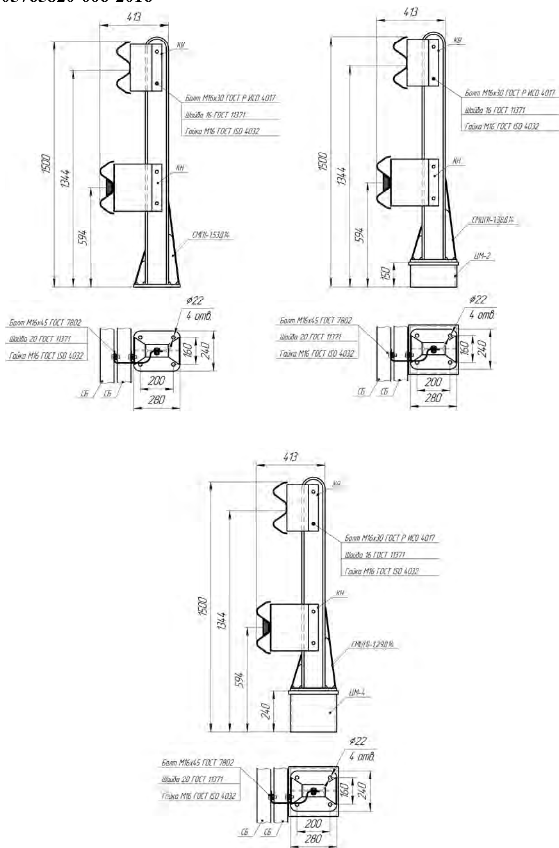
Рисунок В.80 – Мостовое ограждение 21МО/450÷500x1,5xS(D14); 21МО/450÷500x1,5(Ц)xS(D14)
