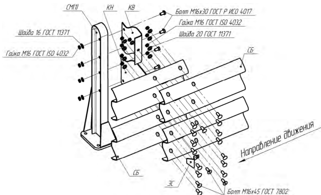
Рисунок В.58 – Схема сборки мостового ограждения 21МО/300÷450-0,9÷1,1
