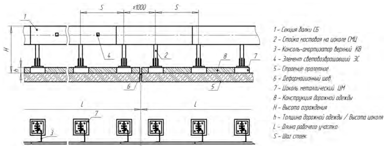
Рисунок В.7 - Ограждение группы 21МО/130-300(Ц)
