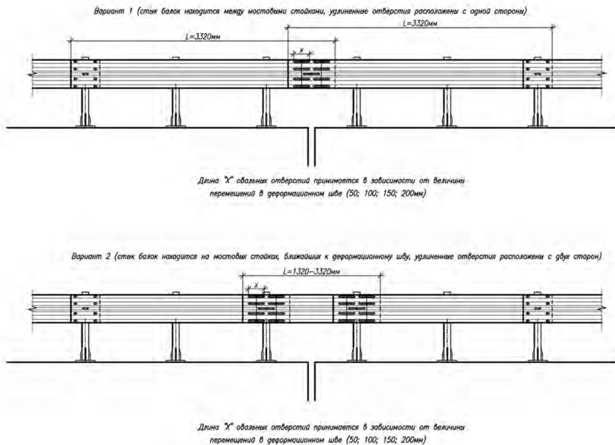
Рисунок В.116 – Схема установки балок СБДШ в зоне деформационных швов при перемещении \leq 200 мм
