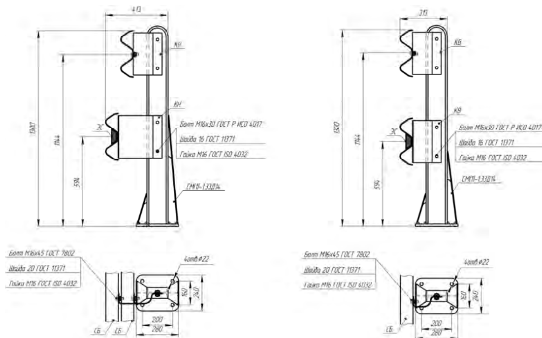
Рисунок В.62 - Мостовое ограждение 21МО/350÷500-1,3хS(Д14); 21МО/350÷500-1,3хS(Д14) без КН
