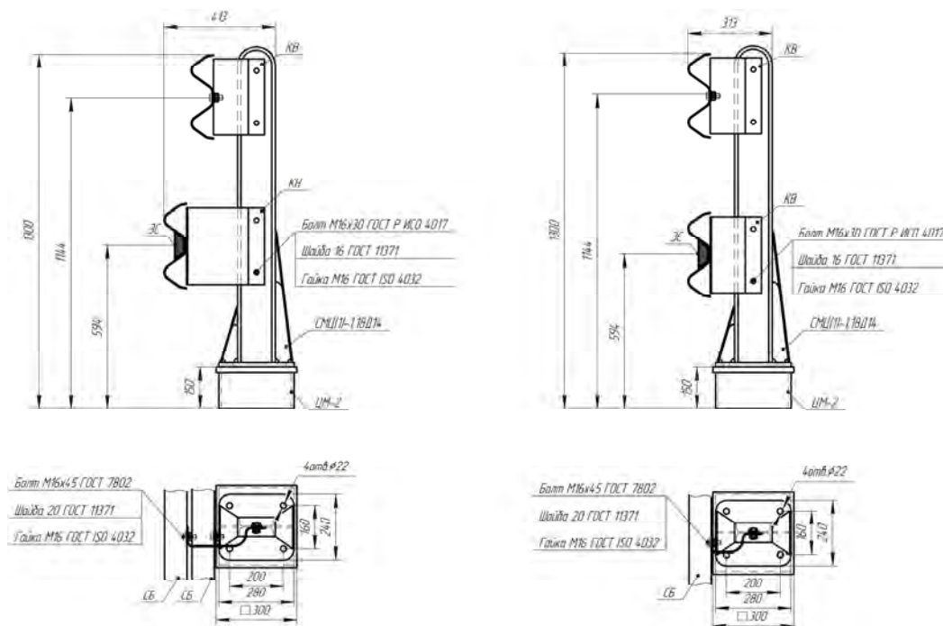
Рисунок В.63 - Мостовое ограждение 21МО/350÷500-1,3(Ц)хS(Д14); 21МО/350÷500-1,3(Ц)хS(Д14) без КН
