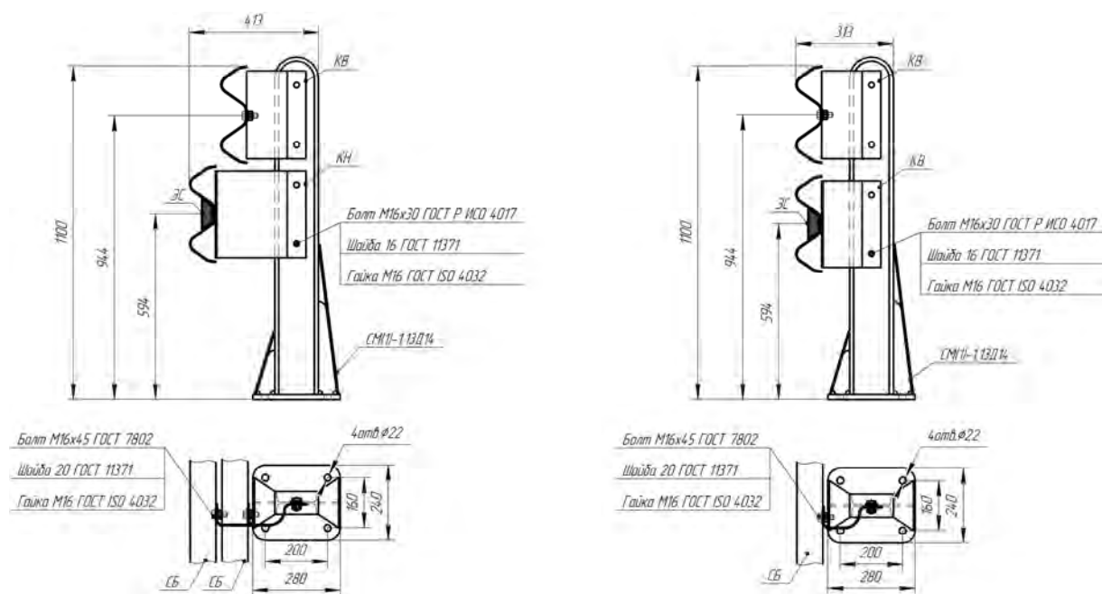
Рисунок В.52 - Мостовое ограждение 21МО/350÷450-1,1xS(D14); 21МО/350÷450-1,1xS(D14) без КН
