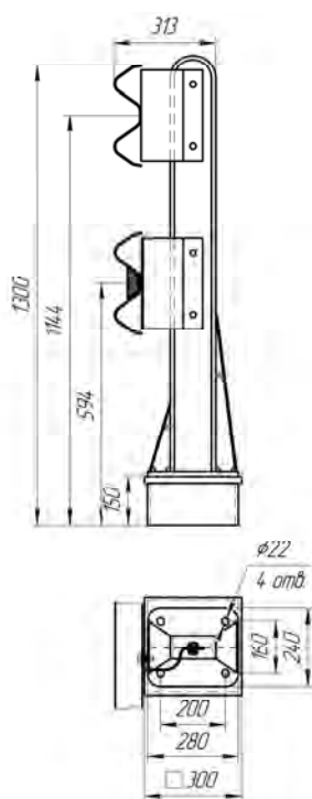
Рисунок 4.70 (СМЦ(1)-1,18Д14) без КН ЦМ-2
