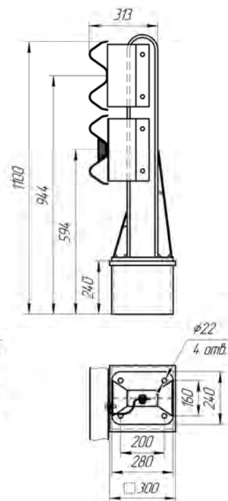
Рисунок 4.61 (СМЦ(1)-0,89Д14) без КН ЦМ-4
