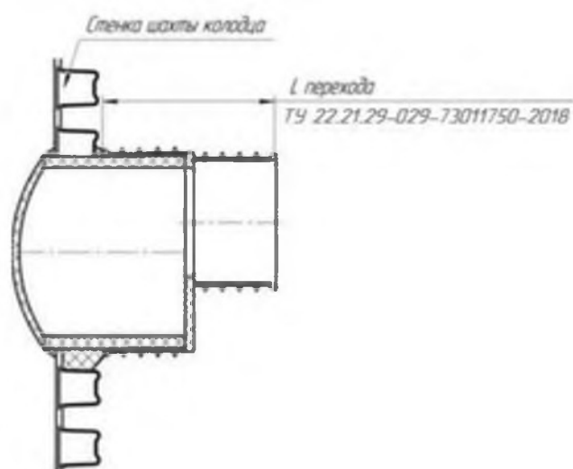
Рисунок 29 – Патрубок с переходом
