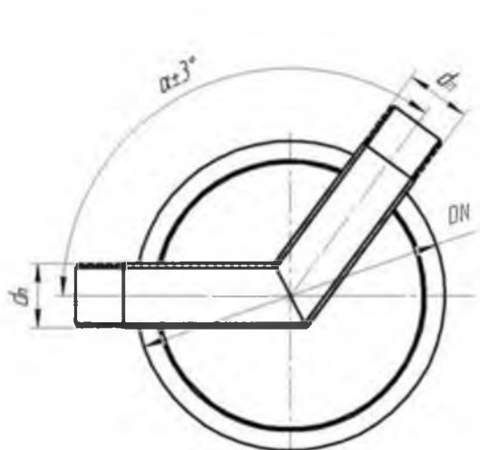
Рисунок 14 – Колодец лотковый угловой
