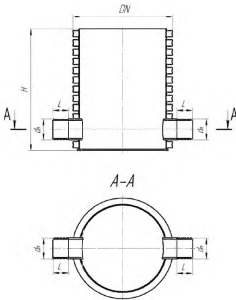
Рисунок 9 – Колодец прямопроходной
