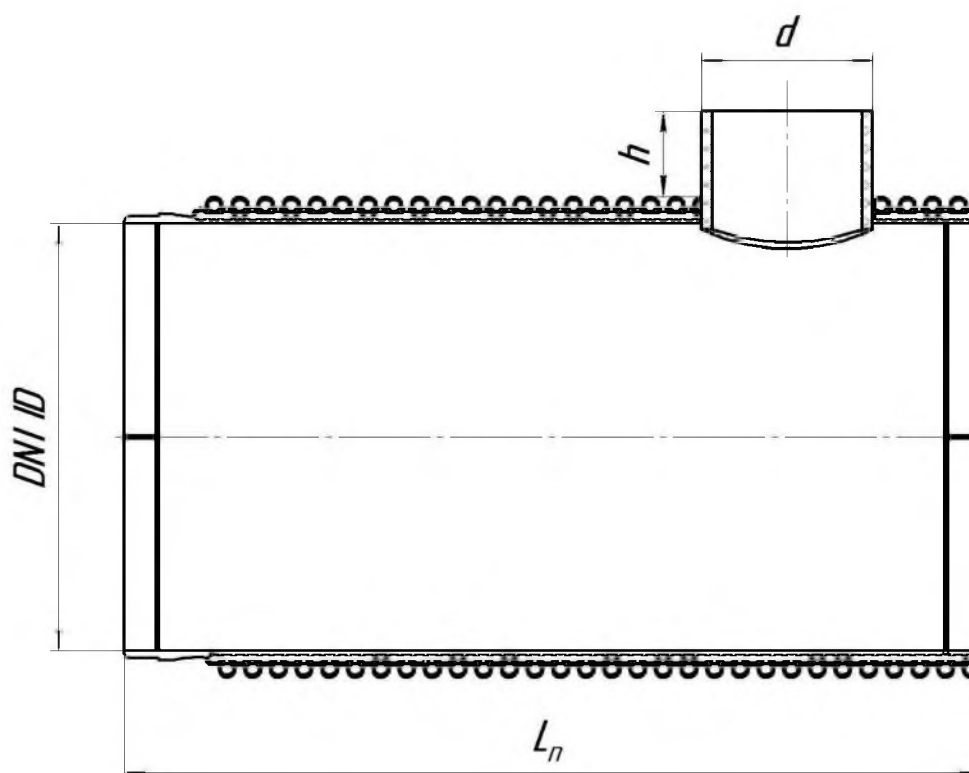
Рисунок 23 – Ёмкость
