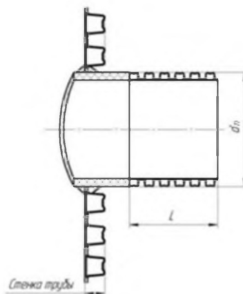
Рисунок 27 – Патрубок трубы со структурированной стенкой
