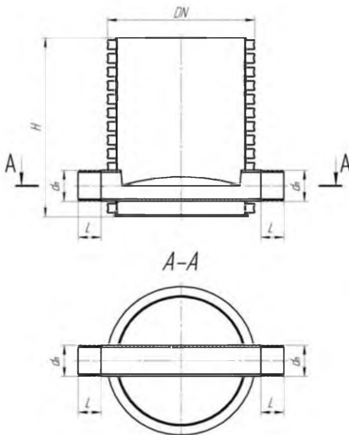
Рисунок 13 – Колодец лотковый прямопроходной
