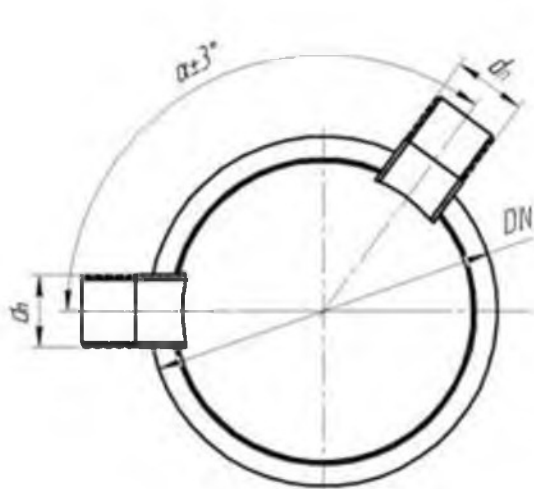
Рисунок 10 – Колодец угловой
