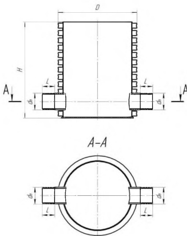
Рисунок 32 – Одноуровневый колодец
