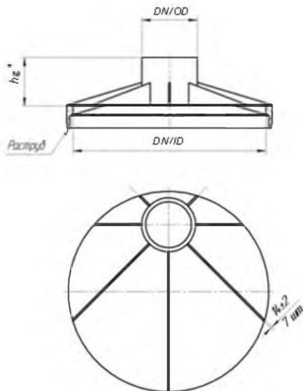
Рисунок 5 – Горловина ПК
