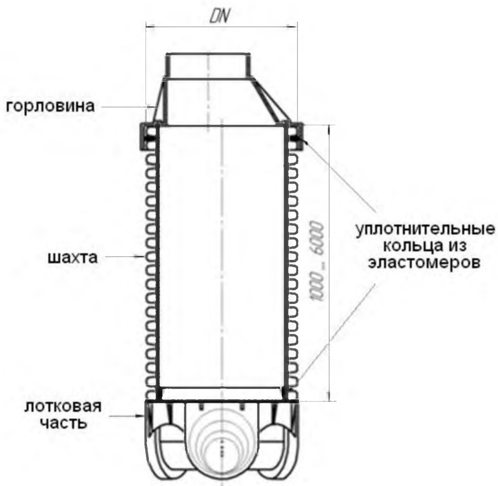
Рисунок 1 – Сборный колодец
