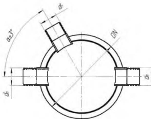
Рисунок 11 – Колодец тройниковый
