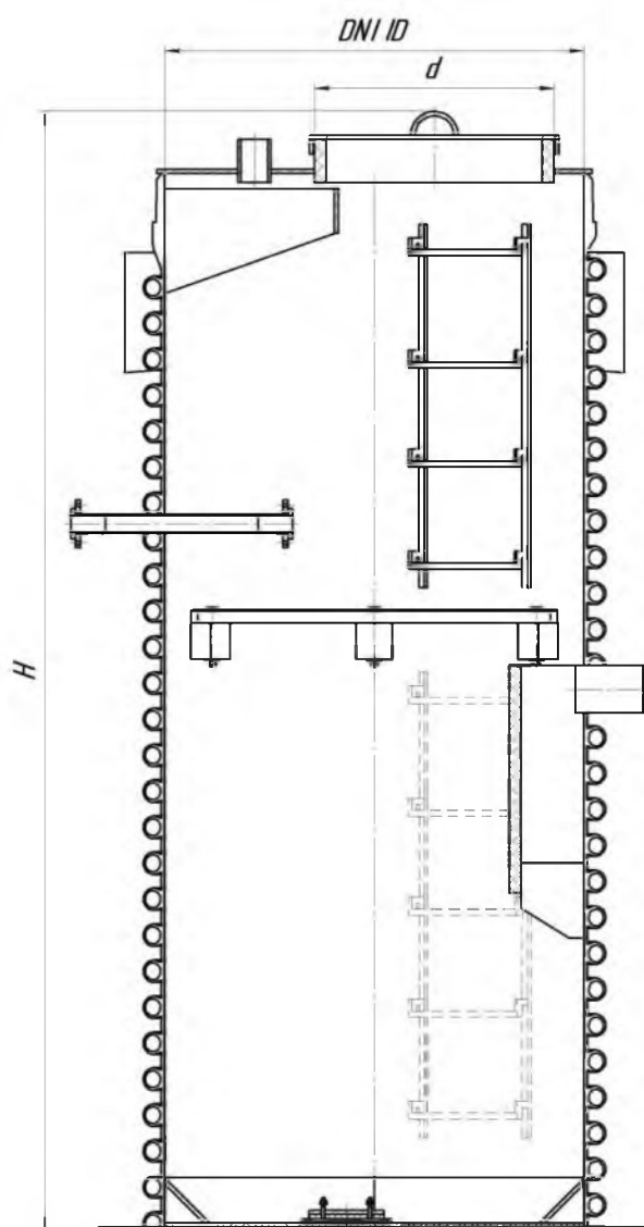
Рисунок 21 – Камера КНС
