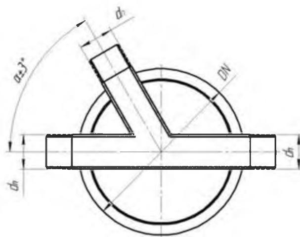
Рисунок 15 – Колодец лотковый тройниковый
