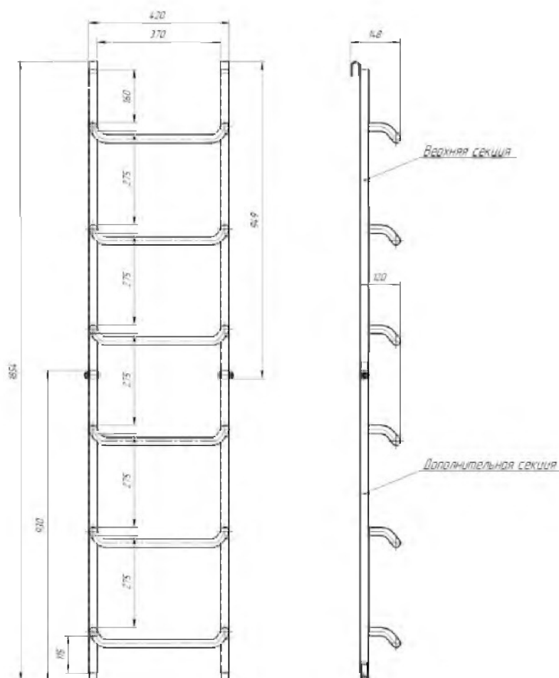
Рисунок 36 – Чертёж лестницы
