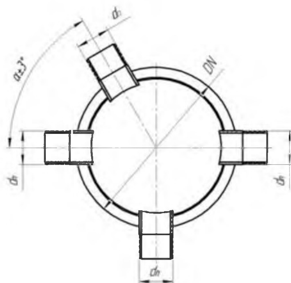
Рисунок 12 – Колодец крестовинный
