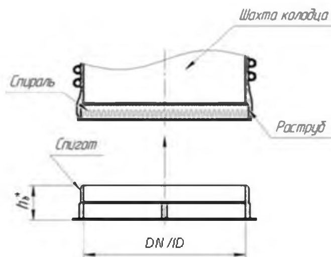
Рисунок 6 – Дно ПК
