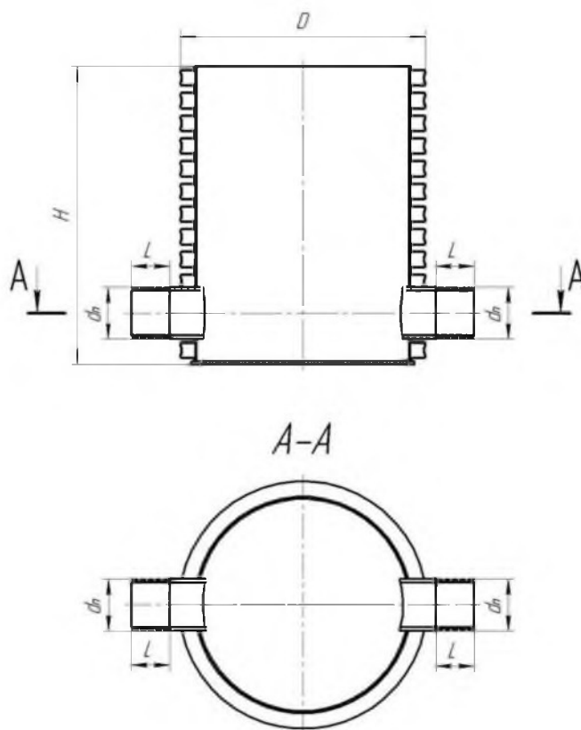
Рисунок 32 – Одноуровневый колодец
