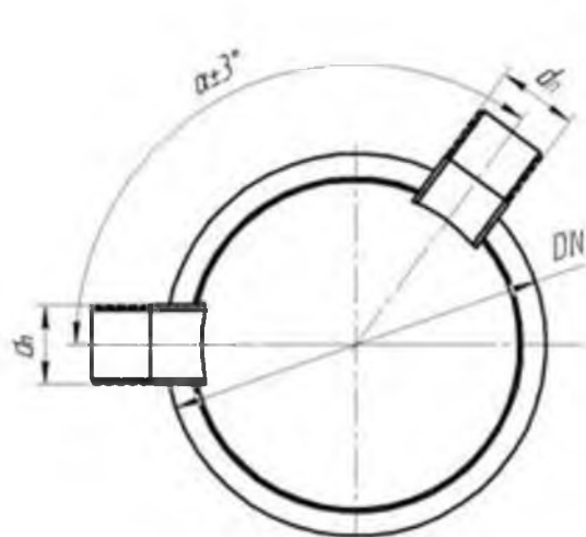
Рисунок 10 – Колодец угловой
