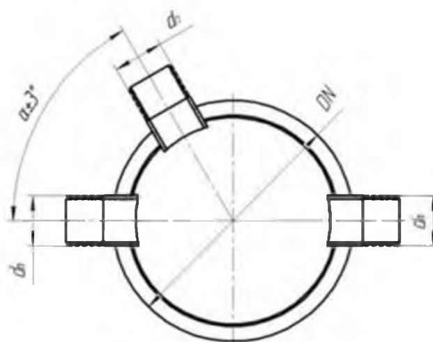
Рисунок 11 – Колодец тройниковый
