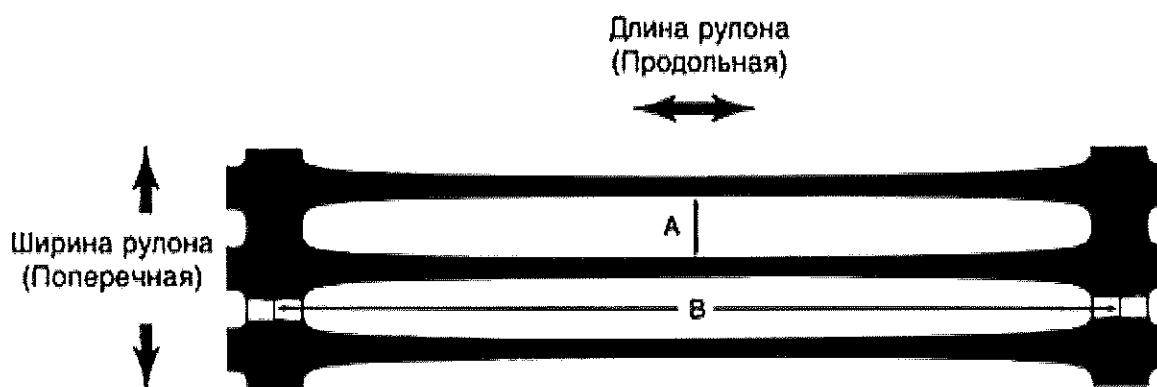
Рисунок А.2 Георешетка марки «Славрос СО»
