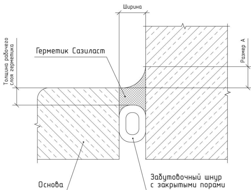
Рисунок 6. Герметизация углового примыкания
