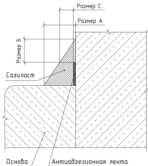
Рисунок 7. Герметизация углового примыкания с использованием антиадгезионной ленты
