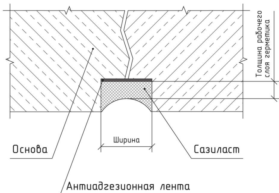
Рисунок 5. Герметизация трещины после предварительного расширения
