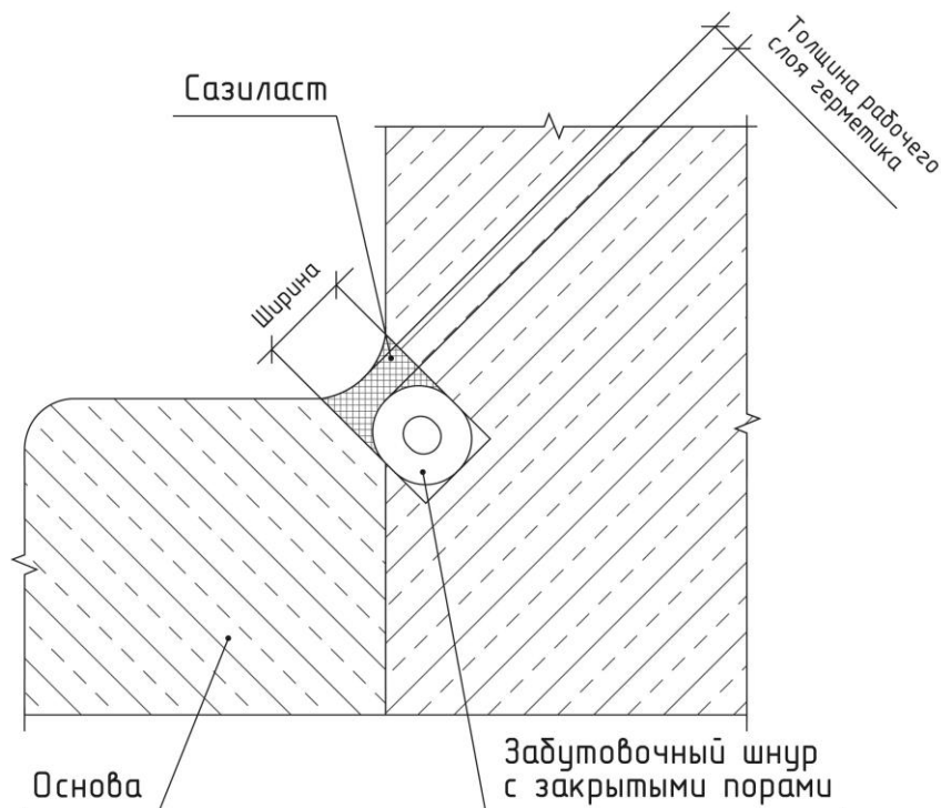
Рисунок 8. Герметизация углового примыкания с использованием антиадгезионной ленты
