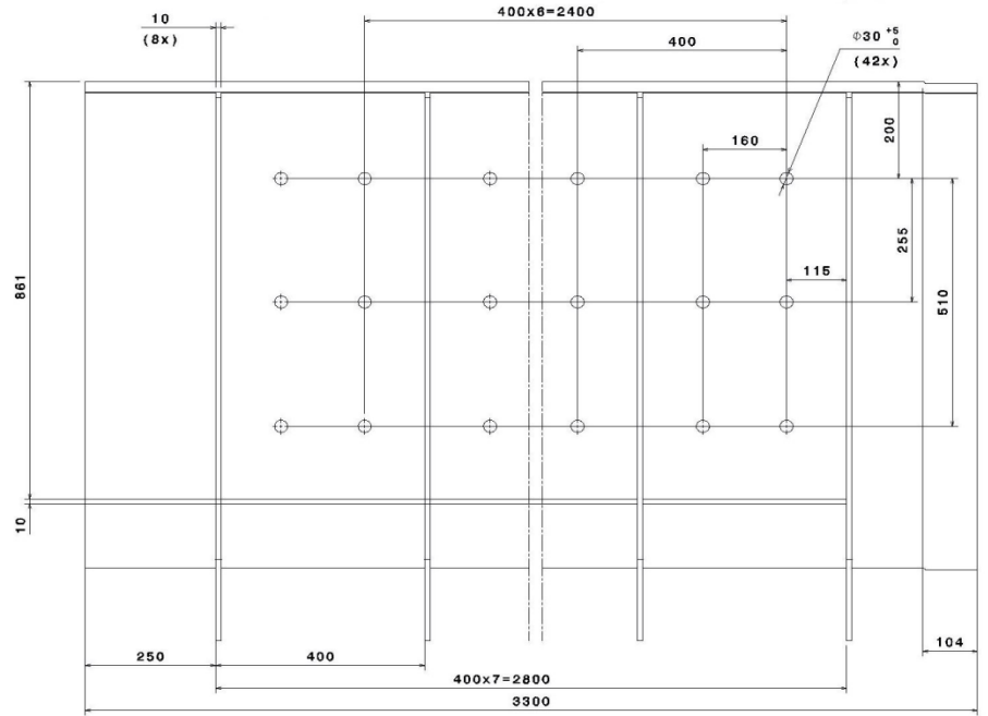
Рис. В1. ВД-0030-1000. Водоотвод железнодорожный. Масса лотка длиной 3,3 м – 120 кг.
