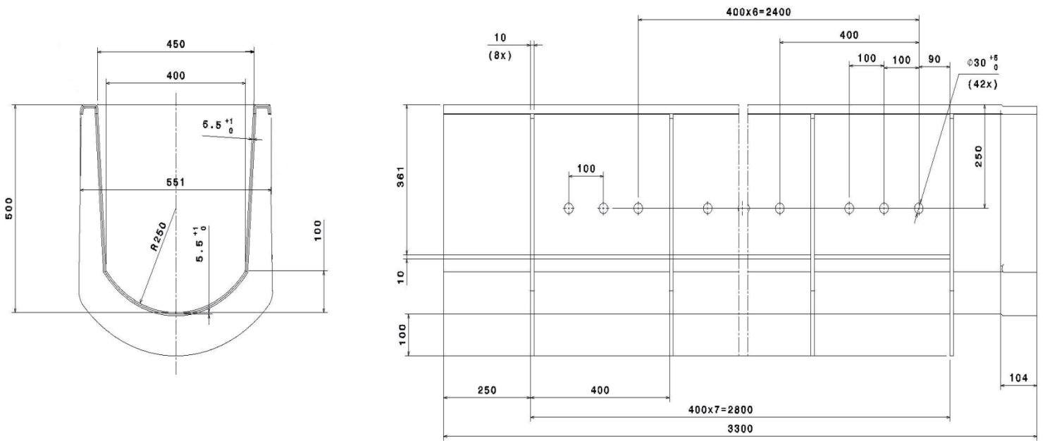
Рис. ВЗ. ВД-0010-500. Водоотвод железнодорожный. Масса лотка длиной 3,3 м – 52 кг.
