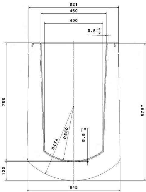
Рис. В1. ВД-0030-1000. Водоотвод железнодорожный. Масса лотка длиной 3,3 м – 120 кг.
