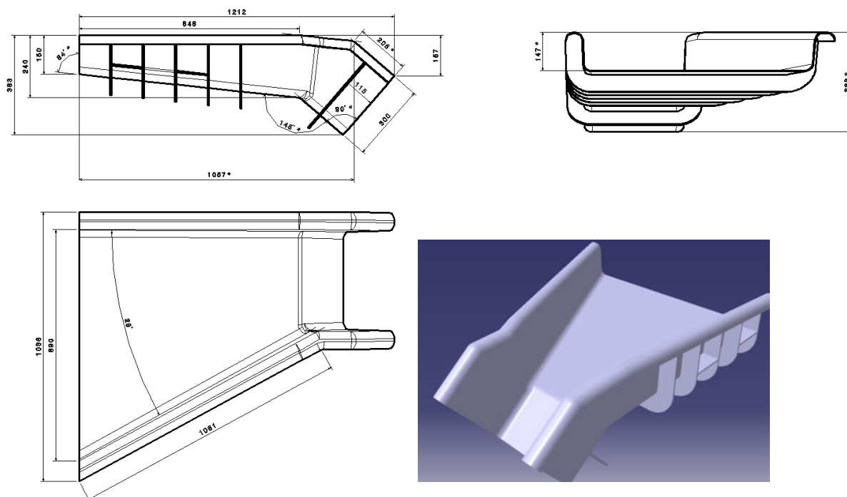
Рис. А6. ВД-005 (ВД-005-1) Быстроток верхний правый (левый – зеркальное отражение) 300х400. Масса – 10 кг
