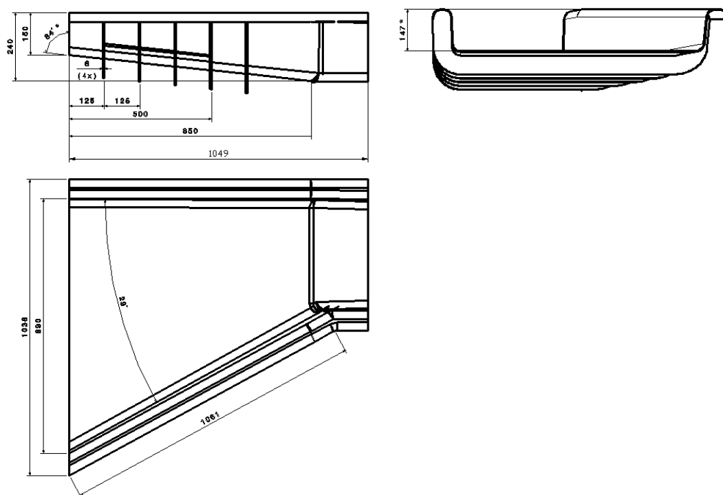
Рис. А7. ВД-005-2 (ВД-005-3) Быстроток верхний правый (левый – зеркальное отражение) прямой 300х400 мм. Масса – 14 кг
