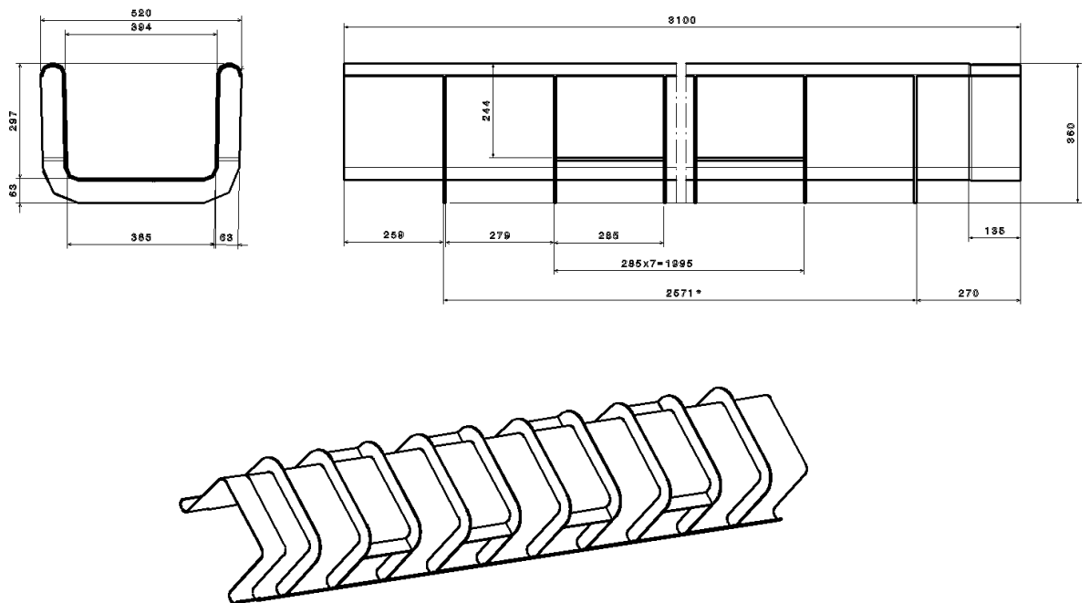
Рис. А1. ВД-003 Быстроток соединительный 300x400. Масса – 23 кг
