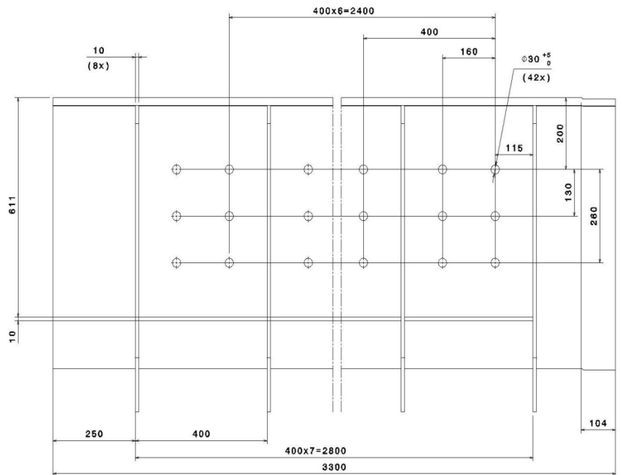
Рис. В2. ВД-0020-750. Водоотвод железнодорожный. Масса лотка длиной 3,3 м – 100 кг.
