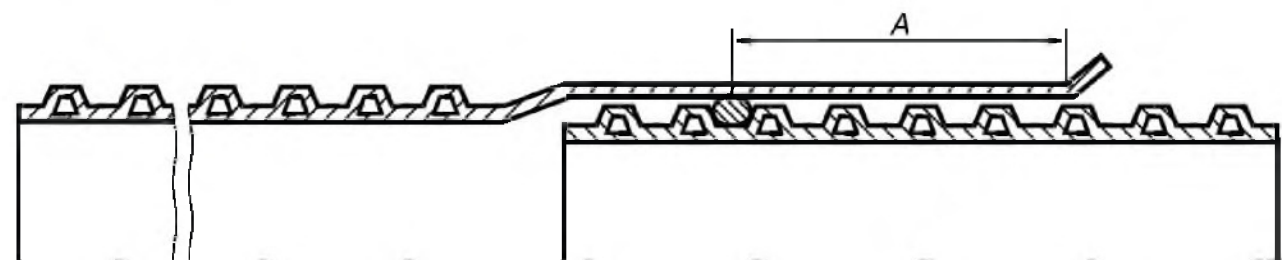
Рисунок 2 – Соединение труб
