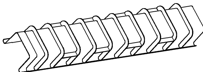
Рис. А1. ВД-003 Быстроток соединительный 300x400. Масса – 33 кг
