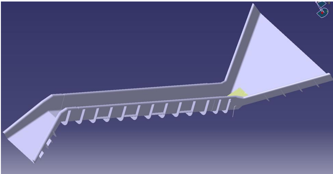
Рис. А12. Водоотвод 300х400 в сборе
