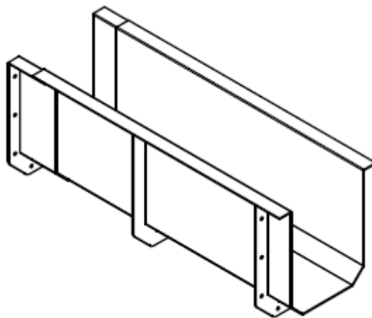
Рис. Д10. ВД-ЛП-2.1 Лоток прямой 290x380 мм. Длина 1,0 м. Возможно изготовление лотков любой меньшей длины по индивидуальному заказу. Масса – 4,5 кг.
