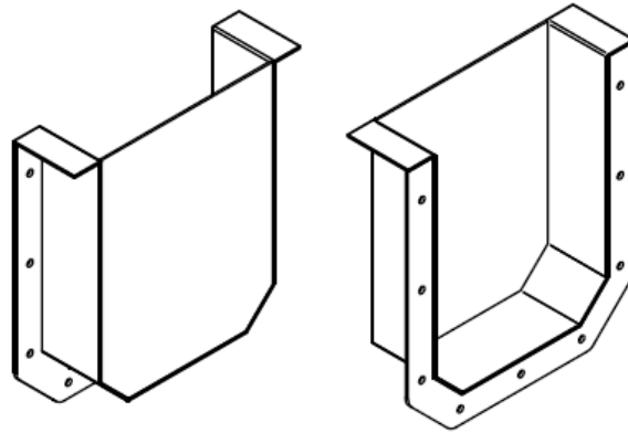
Рис. Д15. ВД-ЛП-7.1. Заглушка 290x380 мм. Устанавливается в начале системы водоотвода. Масса – 1,3 кг.
