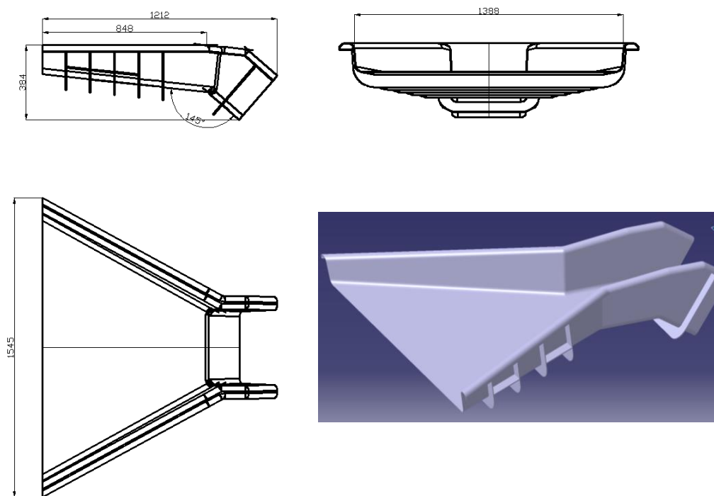
Рис. А2. ВД-004 Быстроток верхний 300x400. Масса – 25 кг
