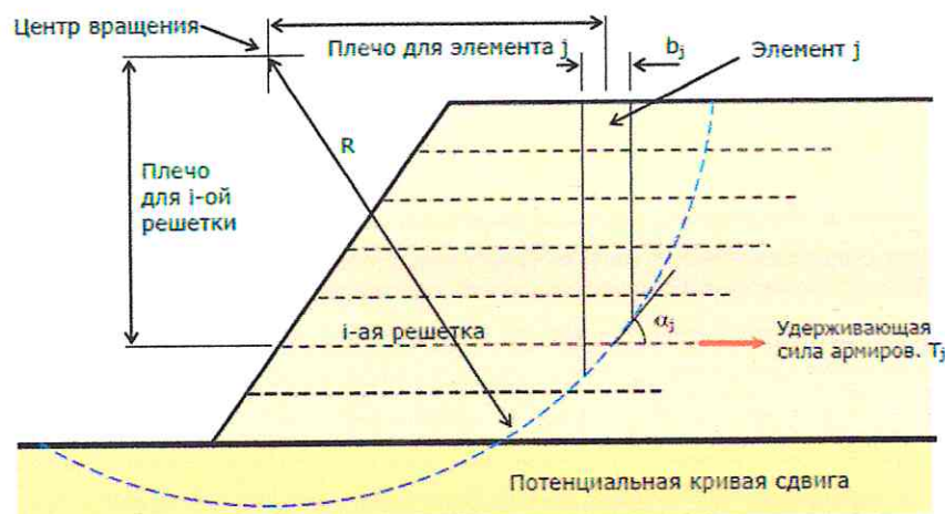
Рисунок А.7 - Цилиндрическая поверхность обрушения
