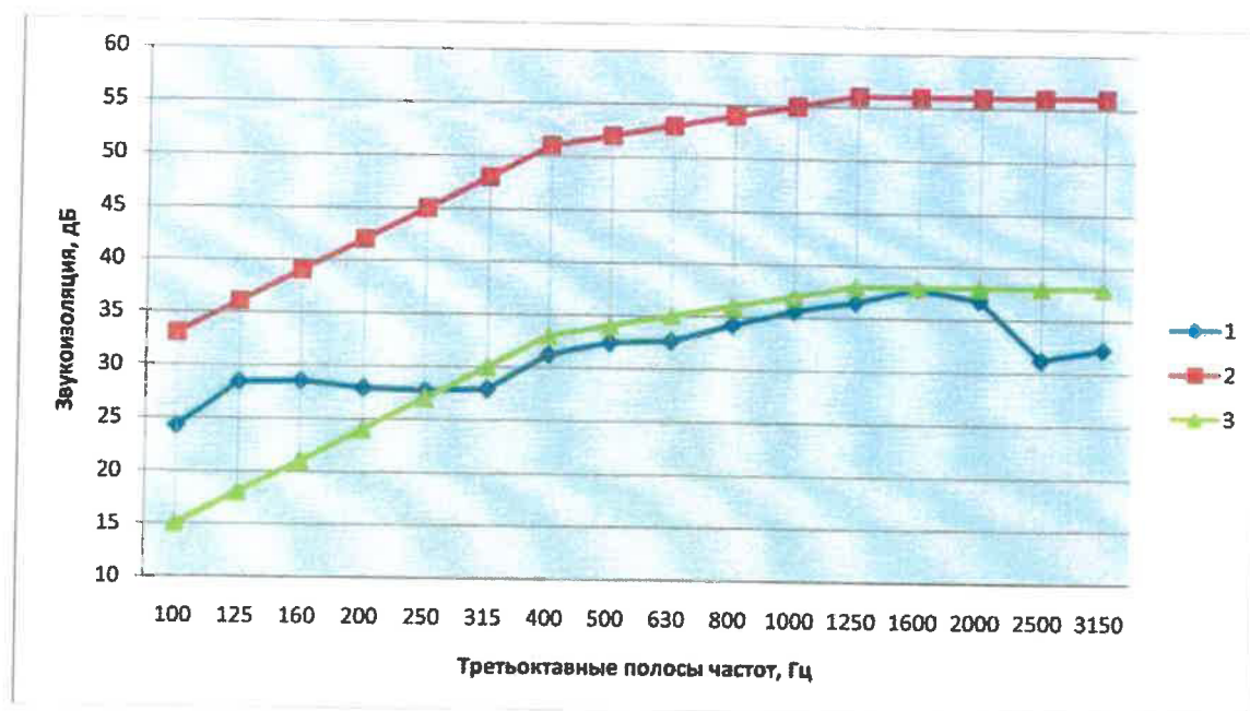
Рисунок 1. Частотные характеристики.
