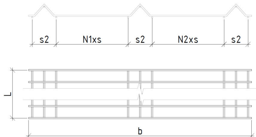
Рисунок В.5 – Вариант исполнения панелей сварных марки «КДП» с тремя ребрами жесткости
