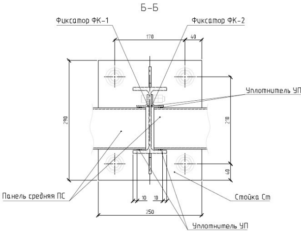
Рисунок А.2 – Сечение А-А и В-В акустического экрана высотой 3 м и шагом стоек 3 м
