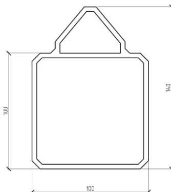
Рисунок 3 – Панель ПН
