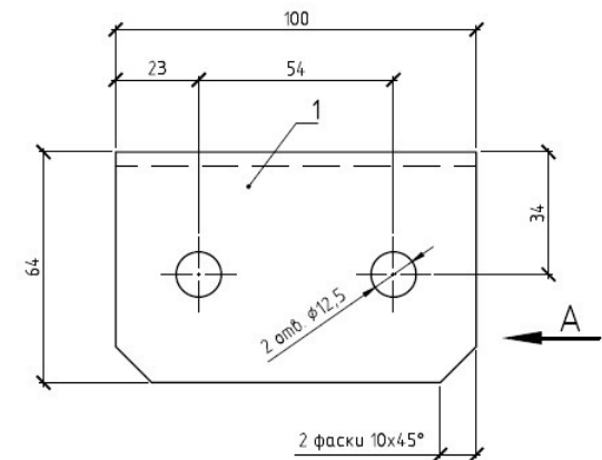
Вид А
