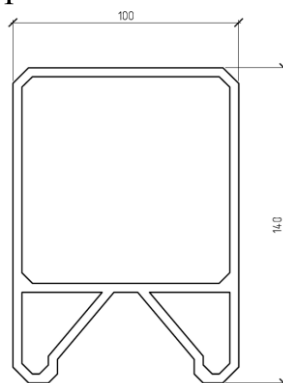
Рисунок 1 – Панель ПВ
