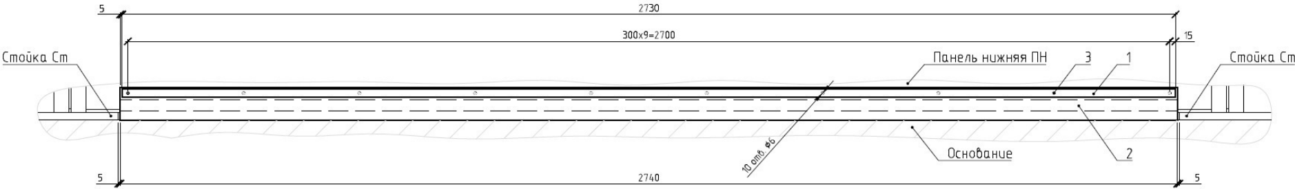
Рисунок А.7 – Крепление нижней Панели акустического экрана высотой 3 м и шагом стоек 3 м
